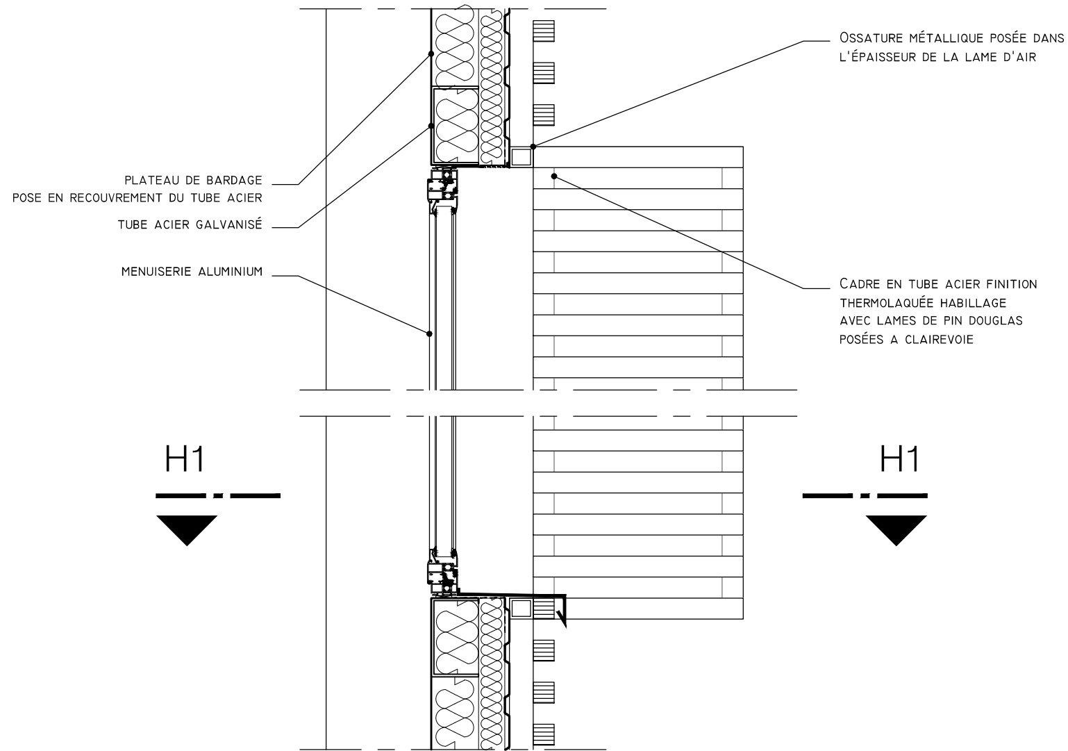
COUPE VERTICALE BRISE-SOLEIL FIXE EN LAME DE BOIS - 1/10°
