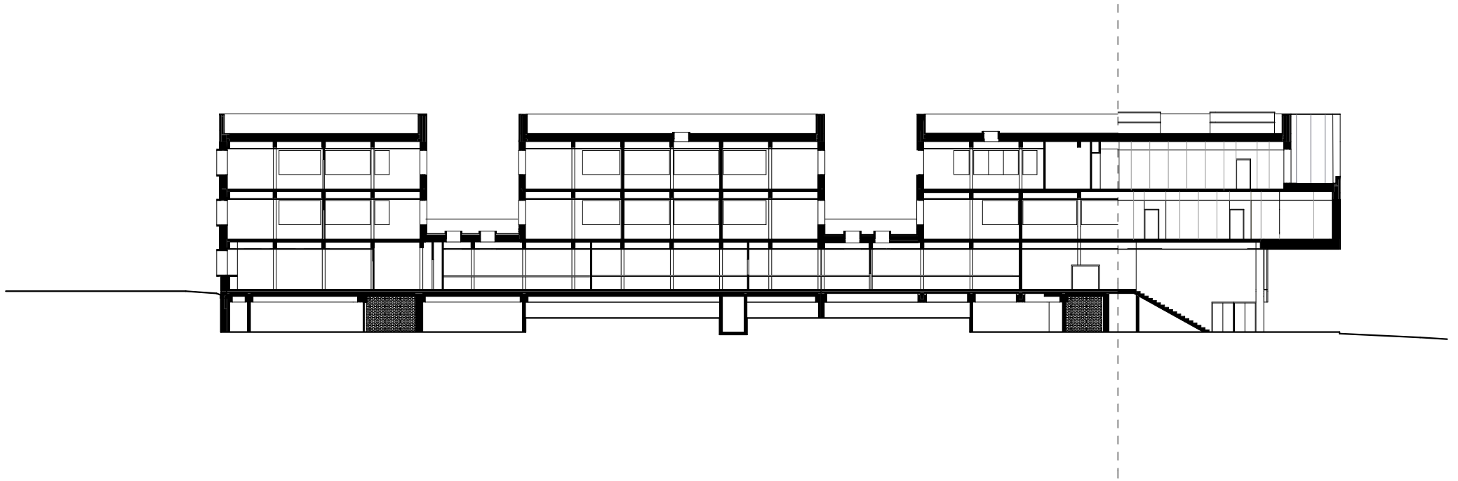
COUPE SUR HALL ET PATIO
