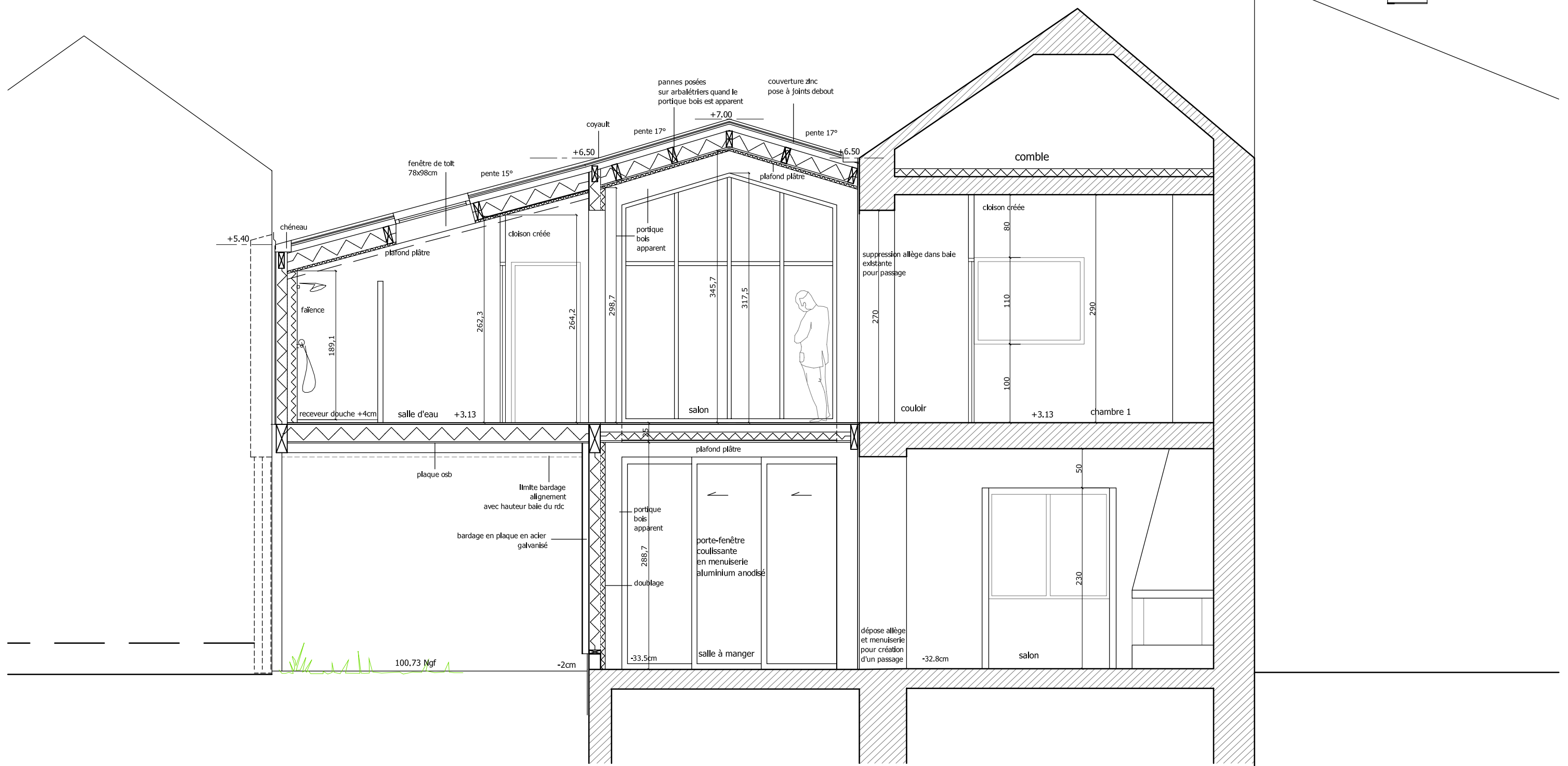
Coupes Nord/Sud Coupe D - 1/50
